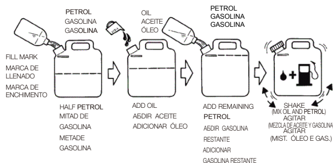
FUEL MIXTURE CHART: TABLA DE MEZCLA DE COMBUSTIBLE: DIAGRAMA DE MISTURA DO COMBUSTÍVEL:
