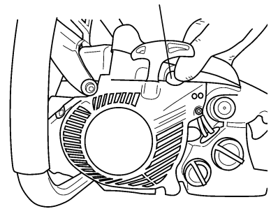
Primer pump Bomba de cebado Bomba de ferragem
